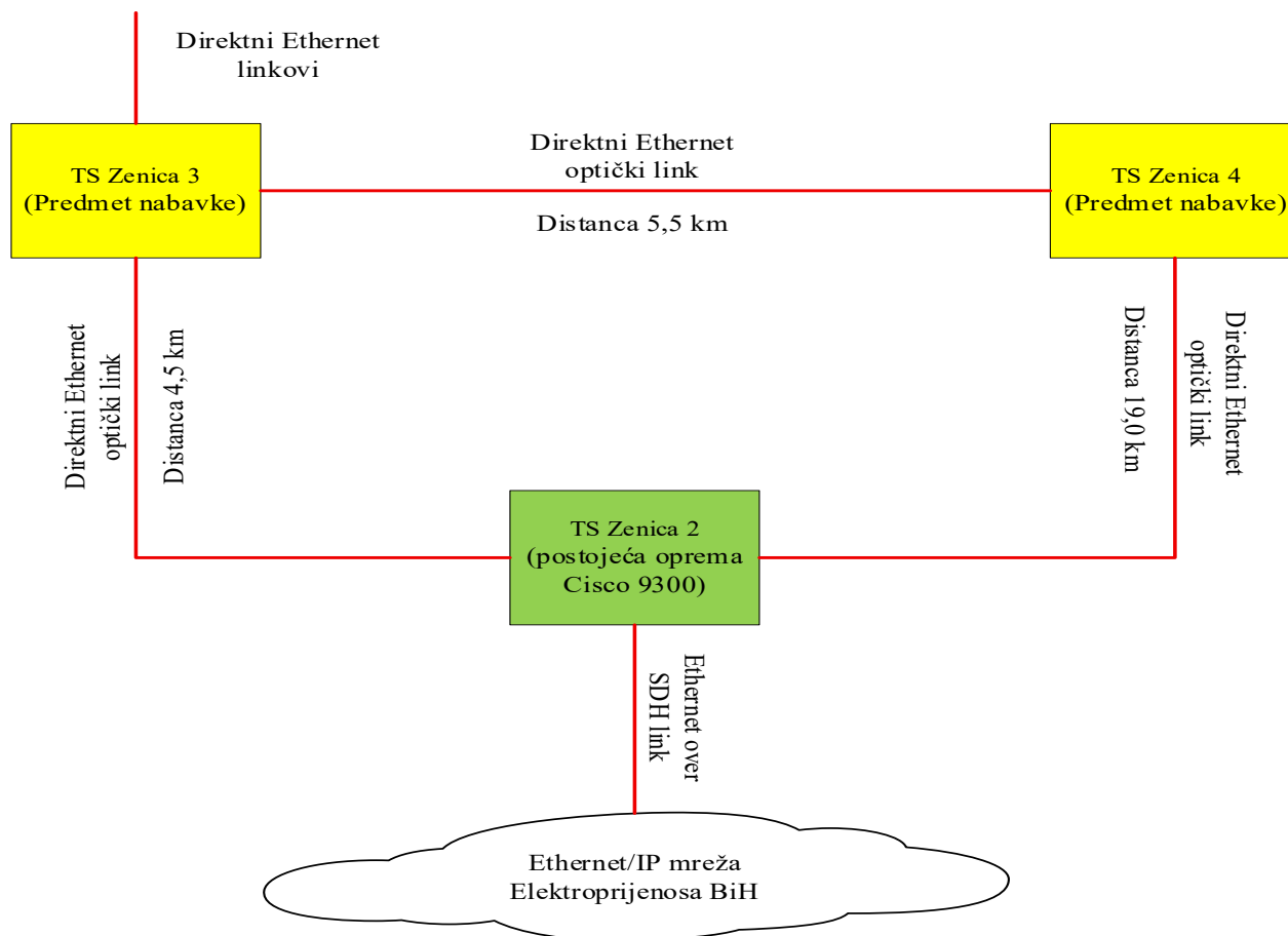
Slika 2.1 – Segment Ethernet/IP mreže koji je potrebno realizovati kroz predmetnu nabavku
