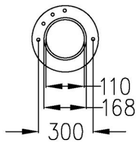
GORNJA FLANSNA 12 RUPA \Phi 14 mm
