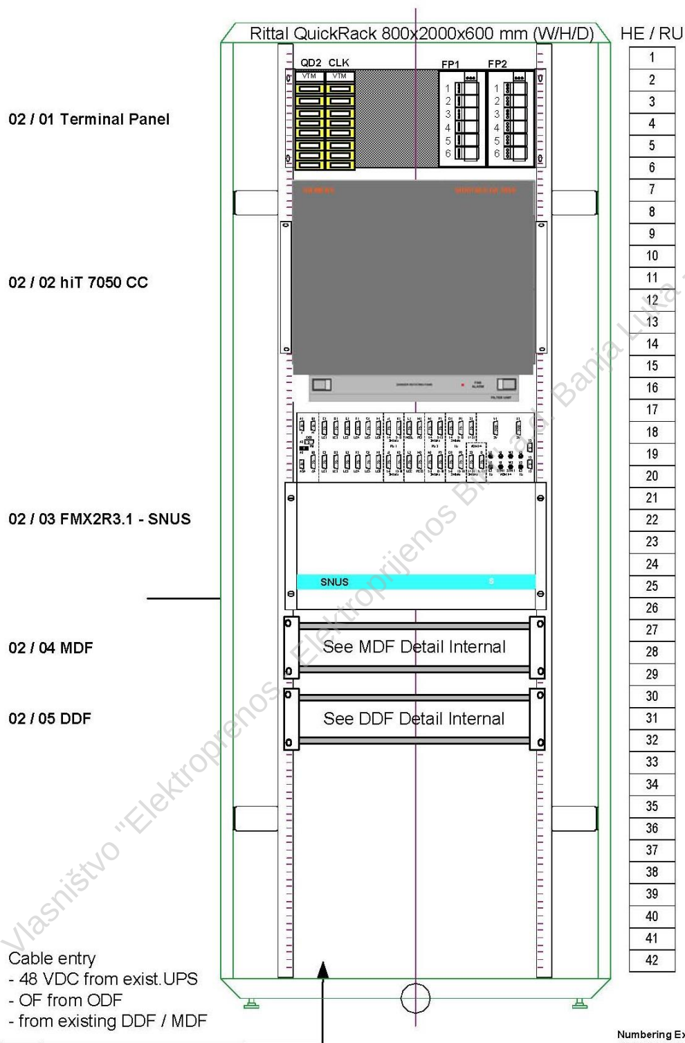
Slika 1.2-Položaj PDH, SBN-a i MDF razdjelnika smještenih u TS 110/x kV Goražde 1
