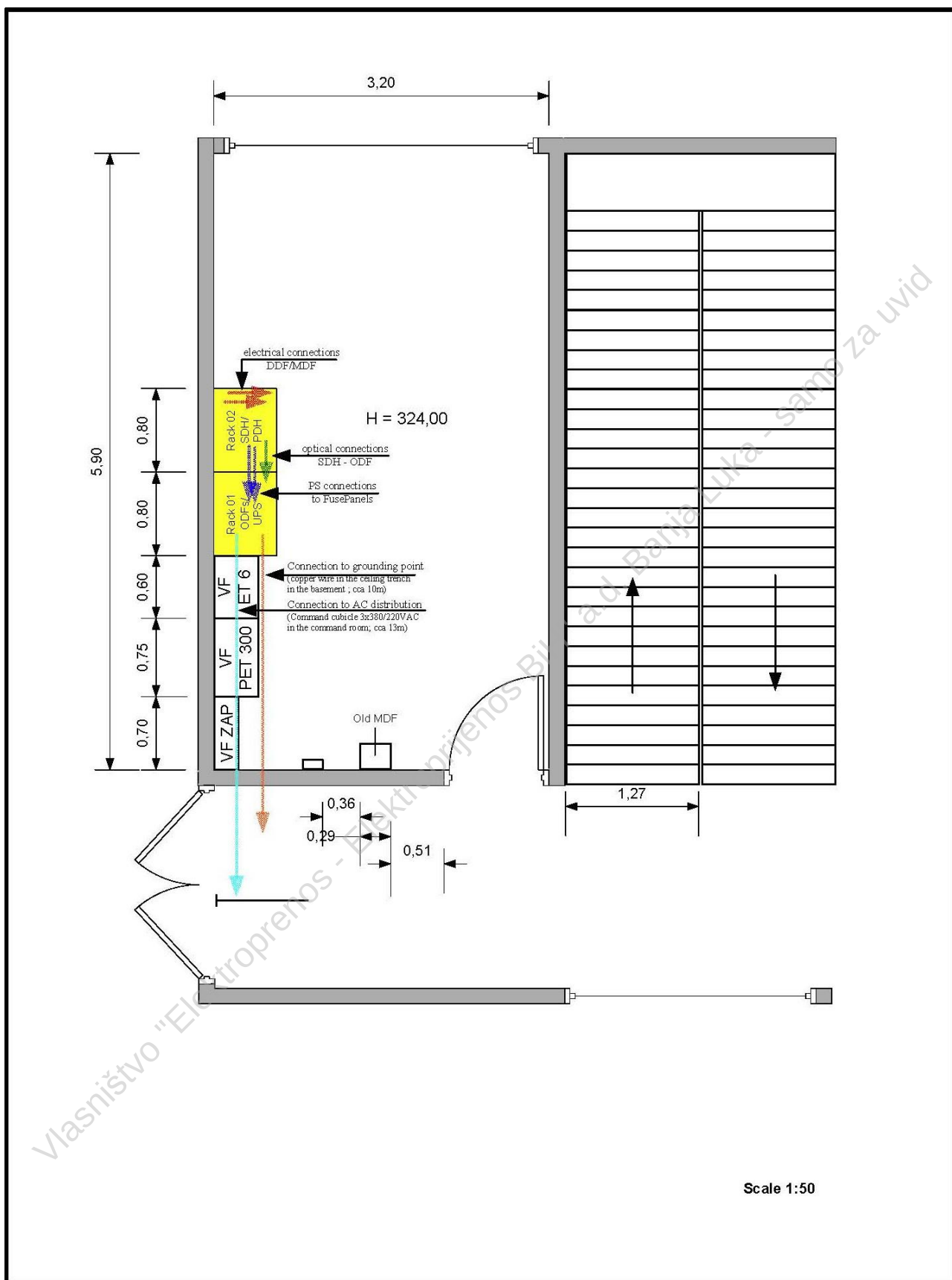
Slika 1.3-Položaj SDH opreme, DDF razdjelnika i ODF-a smještenih u TS 110/x kV Goražde 1
