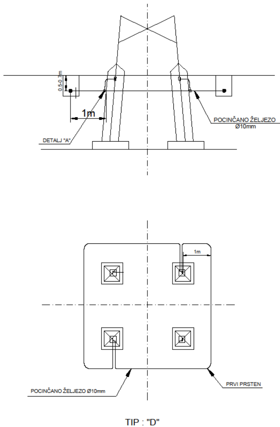
Slika 1. Uzemljivač tipa „D”
