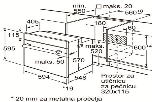
Slika 1: Mjere za ugradbenu rernu
