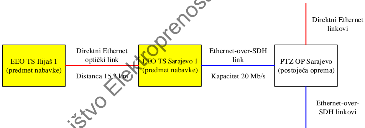
Slika 2.1 – Segment Ethenet/IP mreže koji je potrebno realizovati kroz predmetnu nabavku
