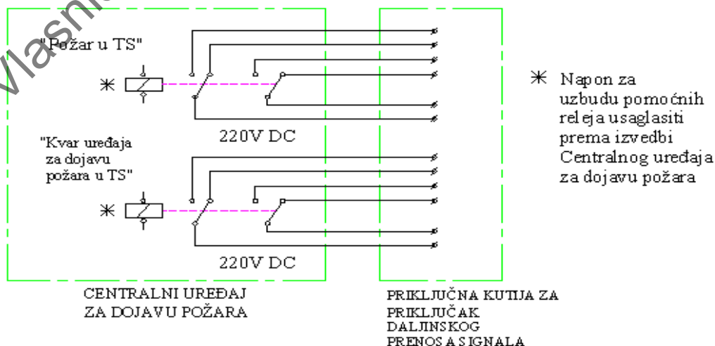
Šema priključaka bezstrujnih preklopnih kontakata iz tačaka a) i b)
