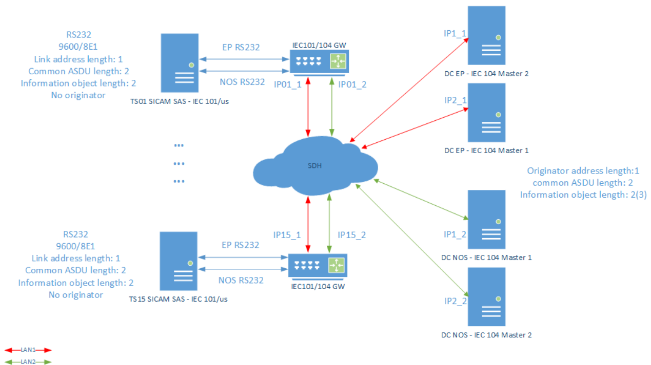
SCADA komunikacije
