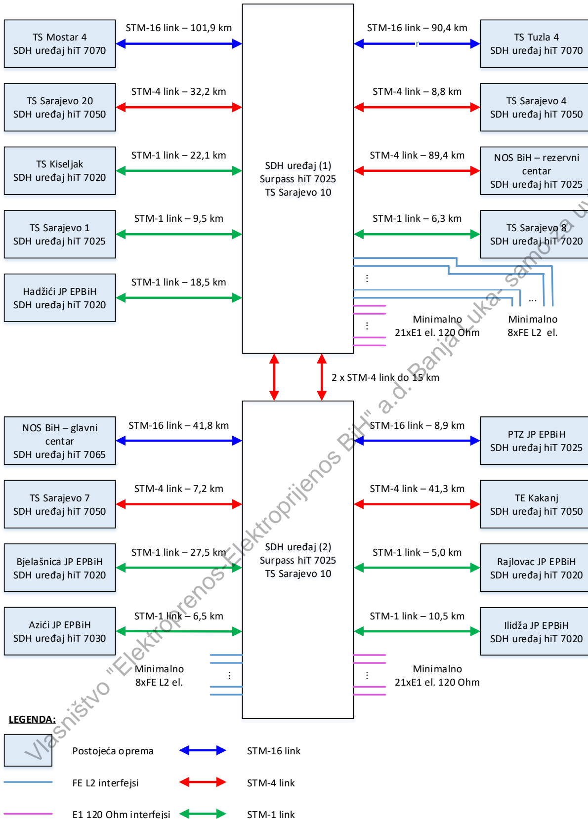
Slika 1. – Segment SDH mreže koji je potrebno realizovati kroz predmetnu nabavku
