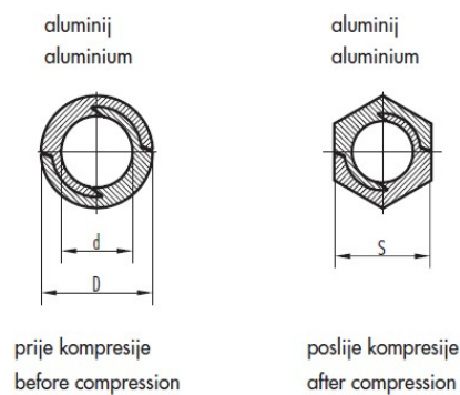
Presjek A-A Section A-A
