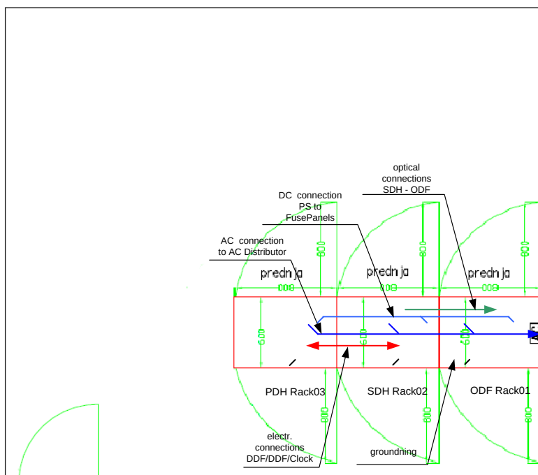
Prikaz postojeće veze između TK ormara kao i napajanja istih
