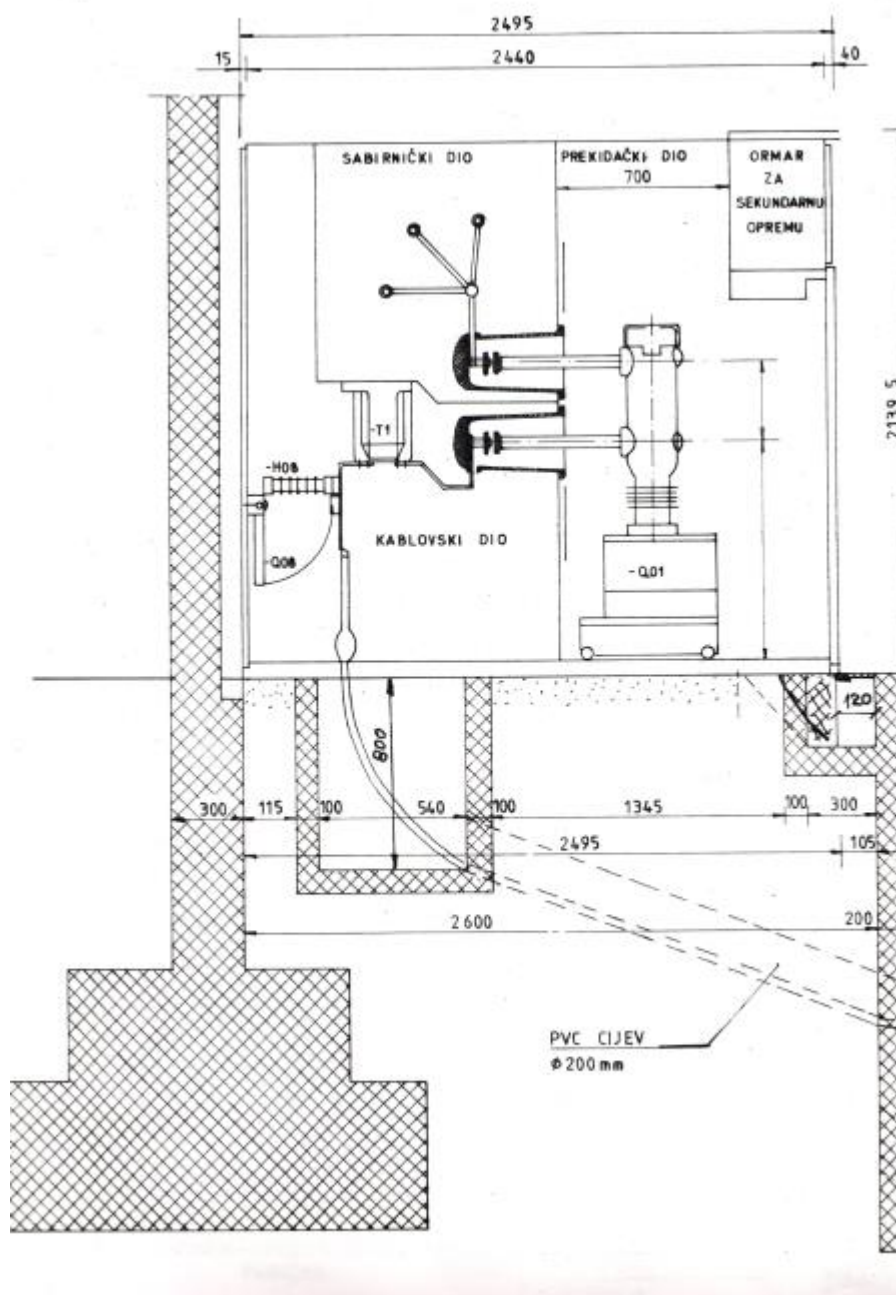
Slika 1.4.7 Presjek odvodne 35 kV ćelije u TS Zenica 4
