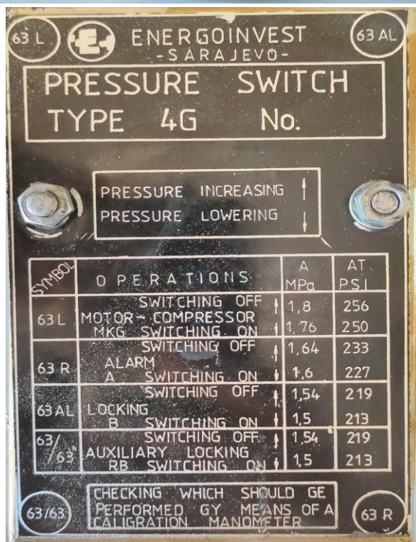
PRILOG 4.5 – Manodenzostat (gore) i presostat (dole) za pogon EPM 255
