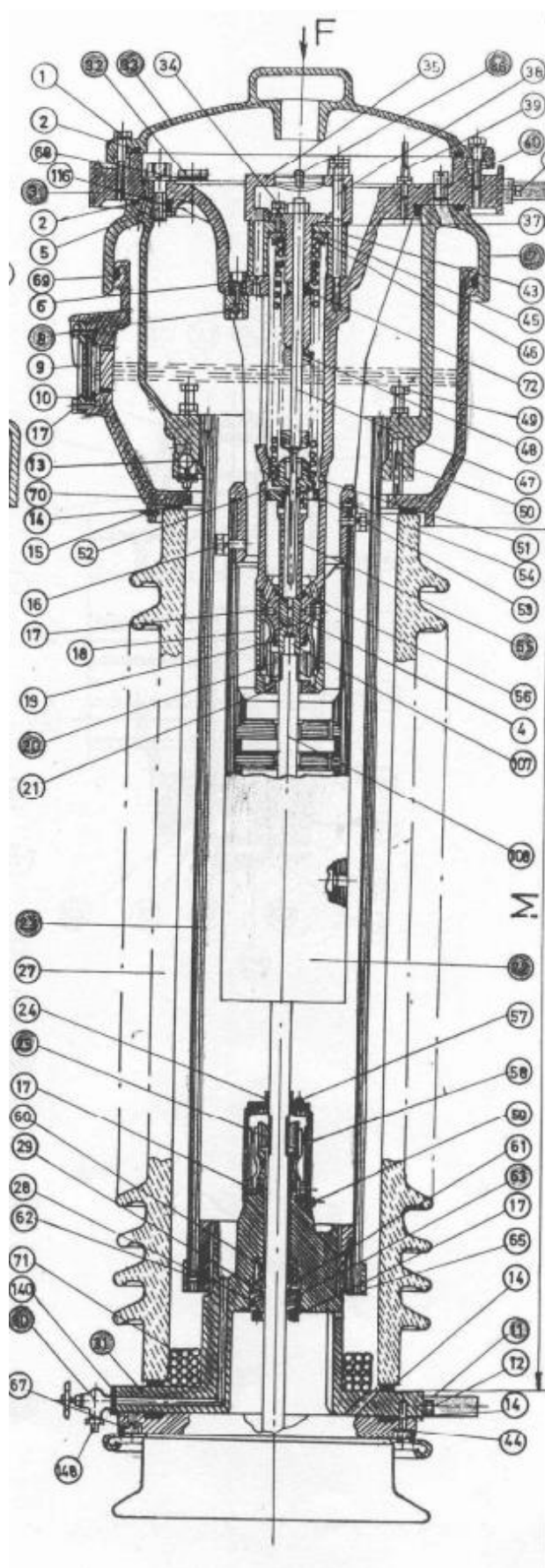
PRILOG 4.10 – Prekidač HPGE
