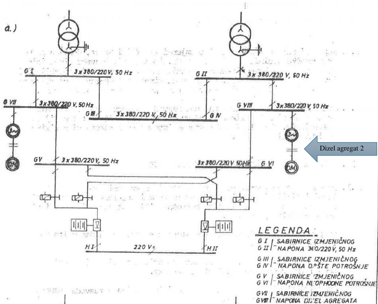
Slika 2. Šema postrojenja vlastite potrošnje
