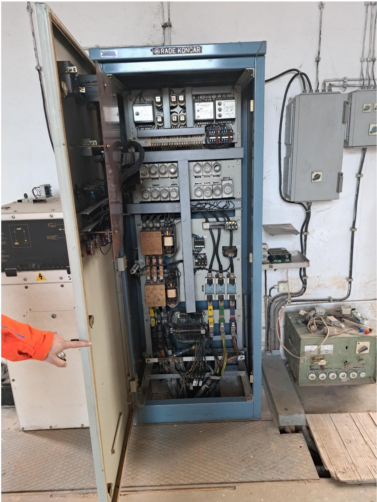
Slika br.3 Komandni ormar dizel električnog agregata
