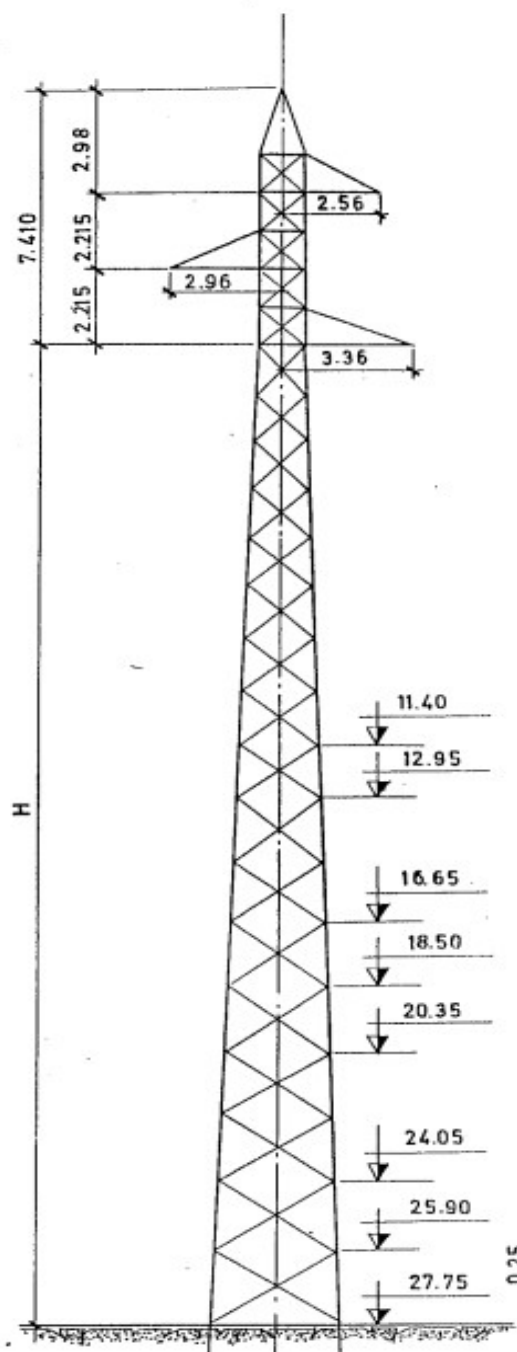
Sl. 1. Silueta nosnog stuba M2
