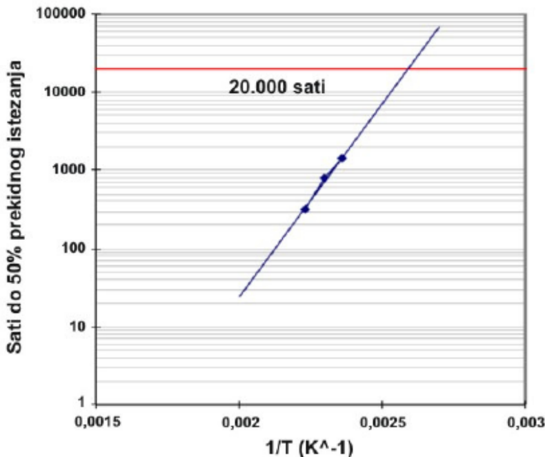
Arheniusov grafik
