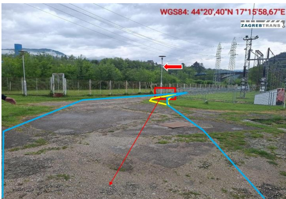
Slika 11- Potrebno ukloniti ivičnjak 1,5m od puta te nasipati, poravnati te zbiti podlogu (60t/m 2 ), potrebno je osigurati put (plava boja) da se sklop težine (91t) ne uruši zbog kanala koji su vidljivi sa slika, staviti čelične ploče ili sl.
