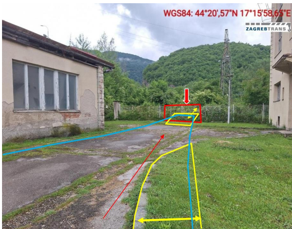
Slika 12- Potrebno je uklanjanje ivičnjaka zbog proširenja, nasuti tampon te izravnati i zbiti, ukloniti ogradu zbog nedovoljnog prostora za dovoz transformatora ( 3,0 m od ograde obezbjediti prostor za manevar), potrebno je provjeriti tlo na kanalima vidljivih sa slike (staviti čelične ploče ili sl.)
